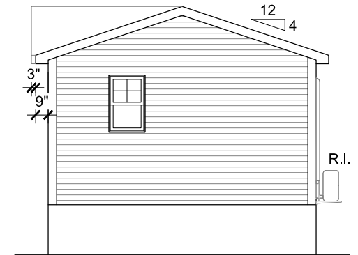
RIGHT ELEVATION
